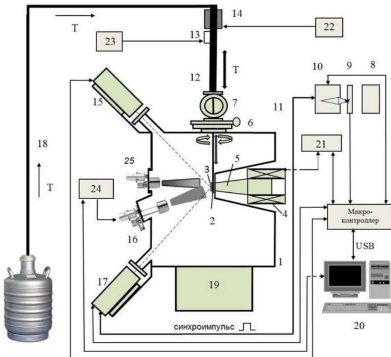
Рисунок 9 – Блок-схема сверхвысоковакуумной многофункциональной установки: 1 – вакуумная камера; 2 – шток с держателем образца; 3 – исследуемый образец; 4 – электромагнит; 5 – магнитопровод; 6 – шиберный затвор; 7 – шлюзовая камера перезагрузки; 8 – источник света; 9 – obtюратор; 10 – монохроматор; 11 – световод; 12 – линейный сильфонный транслятор; 13 – вакуумный сильфонный трёхступенной манипулятор; 14 – проточный испаритель-нагреватель; 15 – блок анализатора; 16 – молекулярный источник; 17 – блок поляризатора; 18 – система подачи азота; 19 – магниторазрядный насос; 20 – компьютер; 21 – блок питания магнита; 22 – блок питания проточного нагревателя; 23 – блок питания нагревателя образца; 24 – блок питания испарителя; 25 – испаритель
