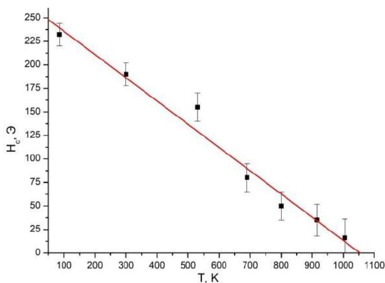
Рисунок 11 – Значения коэрцитивной силы для наноструктуры \text{Fe}/\text{SiO}_2/\text{Si}(100) при нагреве по данным магнитоэллипсометрии
