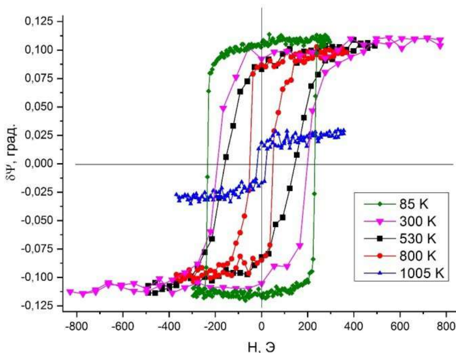
Рисунок 10 – Результаты измерений полевых зависимостей по эллипсометрическому параметру \Psi относительно среднего значения для наноструктуры \text{Fe}/\text{SiO}_2/\text{Si}(100) при различных температурах от 85 до 1005 К
