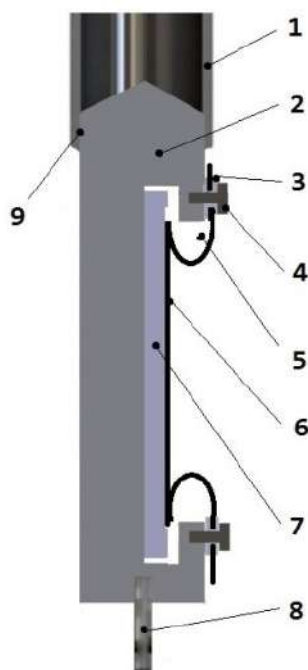
Рисунок 3 – Модель держателя образца в разрезе с элементами для нагрева и охлаждения. Цифрами обозначены: 1 – стальная трубка с хладагентом; 2 – сплошной медный держатель образца; 3 – электроизоляция тоководов; 4 – крепёжные винты; 5 – танталовые тоководы в форме прижимных лапок; 6 – образец (пластина кремния); 7 – пластина сапфира; 8 – фиксатор; 9 – соединение сваркой
