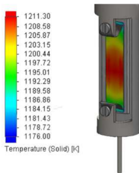
Рисунок 4 – Распределение температуры на подложке при 1200 K
