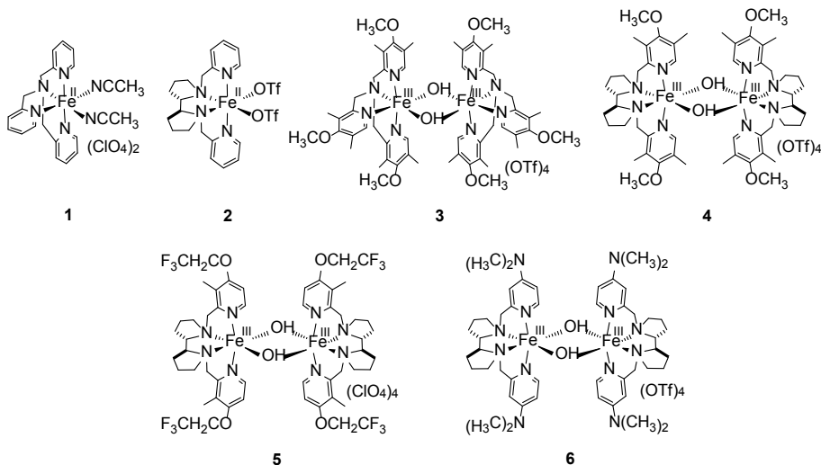
Рисунок 1 – Строение комплексов железа, использованных в работе
