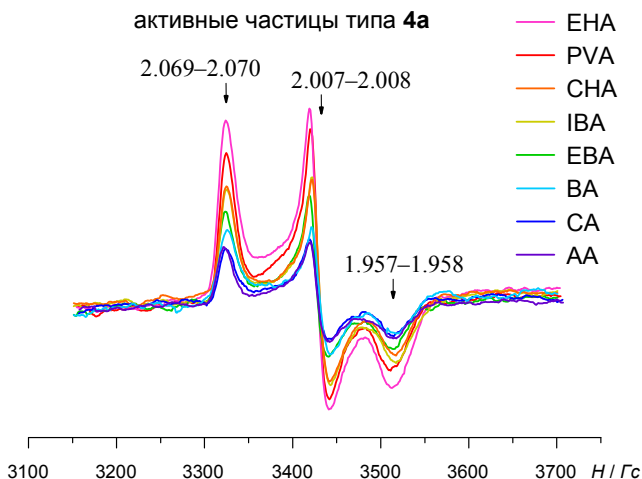
Рисунок 5 – Спектры ЭПР ( -196\text{ }^{\circ}\text{C} ) образцов 4/\text{H}_2\text{O}_2/\text{RCOOH} ( [\text{Fe}]:[\text{H}_2\text{O}_2]:[\text{RCOOH}] = 1:3:10 , [4] = 0.04\text{ M} ), замороженных сразу после смешения реагентов в течение 1.5 мин при -75\text{ }^{\circ}\text{C} в смеси растворителей 1.8:1 \text{CH}_2\text{Cl}_2/\text{CH}_3\text{CN} и выдерживания образцов при -85\text{ }^{\circ}\text{C} в течение нескольких минут для достижения максимума концентрации активных частиц
