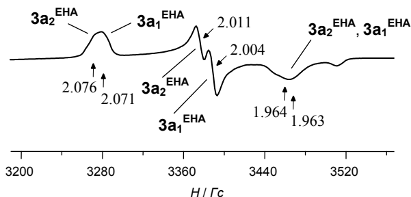
Рисунок 6 – ЭПР спектры ( -196\text{ }^{\circ}\text{C} ) образца 3/\text{CH}_3\text{CO}_3\text{H}/\text{EHA} ( [\text{Fe}]:[\text{CH}_3\text{CO}_3\text{H}]:[\text{EHA}] = 1:3:10 , [\text{Fe}] = 0.04\text{ M} ), замороженного сразу после смешения реагентов в течение 2 мин при -70\text{ }^{\circ}\text{C} . Растворитель – \text{CH}_2\text{Cl}_2/\text{CH}_3\text{CN} ( v/v = 1.8:1 )
