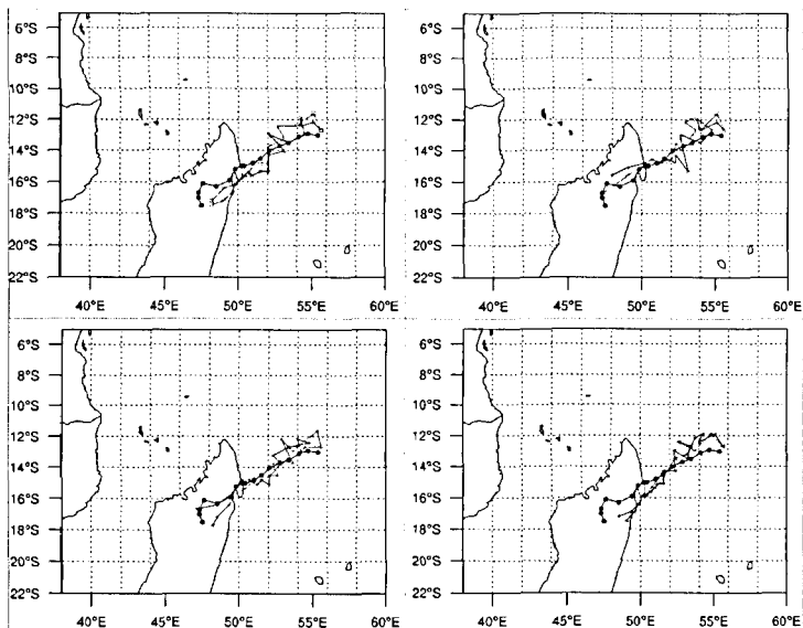
Рисунок 3. Четырехдневный прогноз тропического циклона Jaya с использованием четырёх разных схем микрофизики: а) Lin et б) WSM3 в) WSM5 д) and WSM6, и 1- фактическая траектория; 2-YSU траектория; 3- MJY траектория
