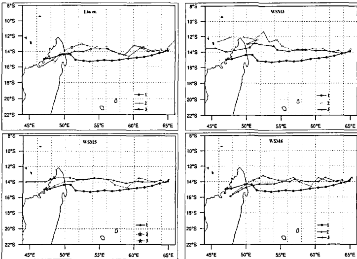
Рисунок 2. Четырёхдневный прогноз тропического циклона Indlala с использованием четырёх разных схем микрофизики: а) Lin et б) WSM3 в) WSM5 д) and WSM6, и 1-фактическая траектория; 2-YSU траектория; 3- MJY траектория.
