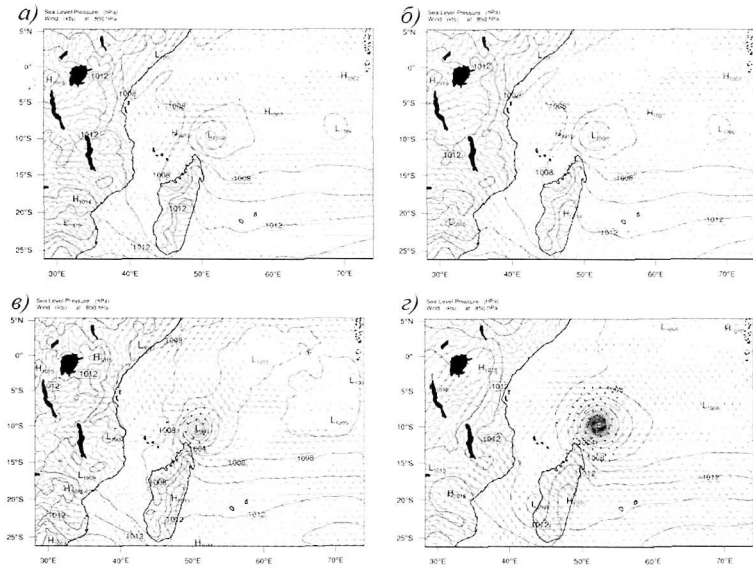
Рис. 4. Горизонтальное распределение давления на уровне моря и поля ветра на уровне 850 гПа в начальный момент времени 1200 UTC 21 Декабря 2006 года для экспериментов а)CTLR б)3DVR в)CYC и д)BDA
