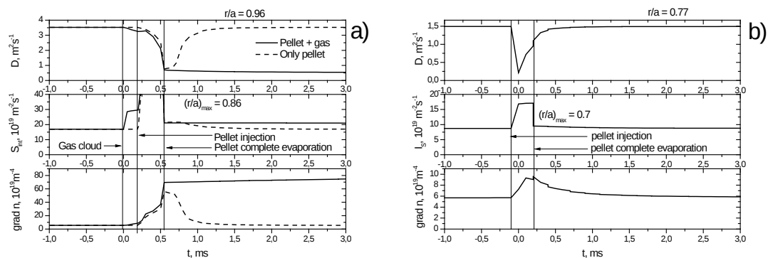
Рис. 5. Результаты моделирования для разрядов с пеллет-инжекцией: L-H переход (a) и кратковременное улучшение удержания (b). На рисунке представлена временная эволюция коэффициента диффузии, интегрального источника частиц и периферийного градиента концентрации. На рис. 5 (a) показана эволюция для экспериментального сценария с пеллетой и облаком газа (сплошные линии) и гипотетического случая аналогичной пеллеты без облака газа (пунктирные линии) [A6].
