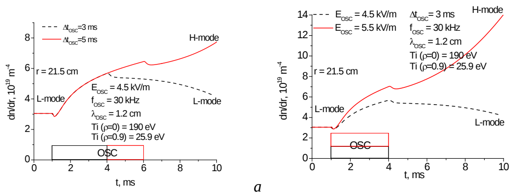
Рис. 1. Результаты моделирования – эволюция периферийного градиента концентрации в токамаке ТУМАН-3М под воздействием возмущения радиального электрического поля при ГАМ: а) вспышки ГАМ разной длительности и б) разной амплитуды. Если длительность (а) или амплитуда (б) вспышки ГАМ превосходят
