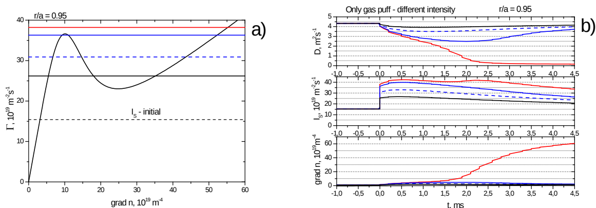
Рис. 7. Зависимость \Gamma(\partial n/\partial r) для разряда в ТУМАН-3М с увеличенным газонапуском без прямого возмущения E_r (а) и результаты моделирования для такого разряда (б). На графике (б) изображена эволюция коэффициента диффузии, интегрального источника и градиента концентрации; цвета линий соответствуют уровням интегрального источника. В случае если интегральный источник лежит выше области трёх пересечений, происходит плавный переход в H-моду [A6].
