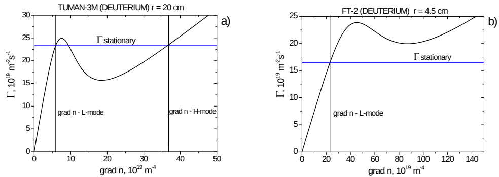
Рис. 2. Зависимость потока частиц от градиента концентрации для разрядов с ГАМ в токамаках ТУМАН-3М (а) и ФТ-2 (б). В сценариях разрядов с ГАМ в токамаке ТУМАН-3М величина источника предполагает два стационарных состояния, L- и H-моду, с возможностью бифуркации удержания. В ФТ-2 для обоих изотопов возможна только стационарная L-мода [A9].
