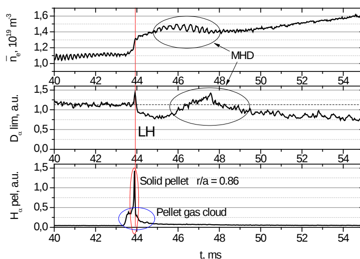
Рис. 3. L-H переход, инициированный пеллет-инжекцией в ТУМАН-3М. Сверху вниз приведены концентрация плазмы, свечение линии D_\alpha на лимитере и свечение линии H_\alpha из области испарения пеллеты. Видна сложная кривая испарения: пик от твёрдого осколка и пологая кривая от сопутствующего газа. Н-мода, характеризующаяся ростом концентрации и спадом линии свечения D_\alpha на периферии, продолжает существовать после испарения пеллеты [A6].
