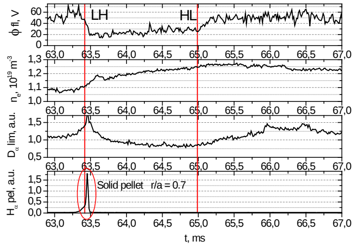
Рис. 4. Временное улучшение удержания при инжекции пеллеты в ТУМАН-3М в результате инжекции твёрдой пеллеты без облака газа и снега от разрушенной части пеллеты. Сверху вниз приведены плавающий потенциал на периферии, концентрация плазмы, свечение линии D_\alpha на лимитере и свечение линии H_\alpha из области испарения пеллеты. L-H и H-L-переходы отмечены вертикальными линиями. Состояние непосредственно после испарения пеллеты обладает характеристиками H-моды (спад свечения периферийной D_\alpha и плавающего потенциала, рост концентрации), однако обратный переход спонтанно происходит через примерно 1.5 мс [A6].
