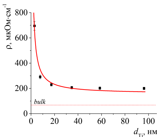
Рисунок 3. Экспериментально измеренные зависимости удельного электросопротивления \rho от толщины напыляемых титановых пленок d_{\text{Ti}} .
