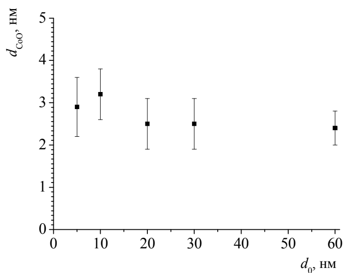
Рисунок 11. Зависимость толщины оксидного слоя d_{\text{окс}} от исходной толщины кобальтовой пленки d_0 .
