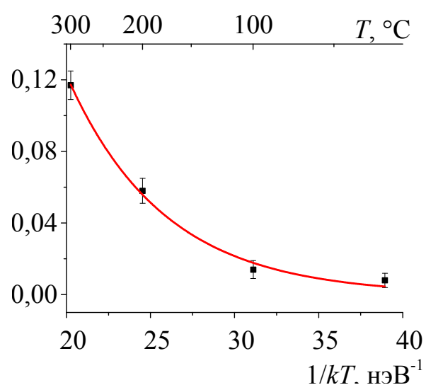
Рисунок 6. Зависимость скорости окисления v_{окс} на воздухе пленки Ti толщиной 20 нм от температуры.
