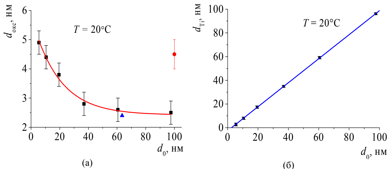
Рисунок 2. Зависимости толщины оксидного слоя d_{\text{окс}} (а) и толщины неокисленного слоя титана d_{\text{Ti}} (б) в бислойной структуре Ti/TiO 2 от исходной толщины окисляемой титановой пленки d_0 . Цветными символами на рис. 2 (а) обозначены толщины оксидных слоев, полученных при окислении: \blacktriangle – пленки ультрачистого Ti толщиной 63.5 нм [10]; \bullet – пленки Ti толщиной 100 нм [11].
