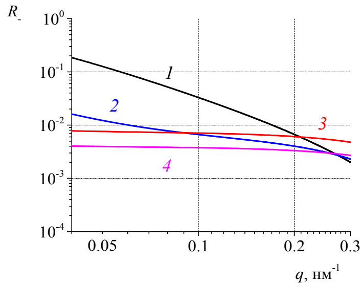
Рисунок 10. Расчетные зависимости коэффициентов отражения нейтронов R(q) от поляризующего зеркала со слоем оксида \text{CoFeO}_x 3.1 нм (1), с бислоем \text{Ti/TiO}_2 6.9/4.0 нм (2), \text{Co/CoO} 7.3/2.9 нм (3) и \text{Co/TiO}_2 5.7/4.0 нм (4).
