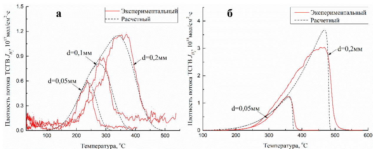
Рисунок 10. Экспериментальные и расчетные зависимости плотности потока водорода термостимулированного газовыделения из пластинок а) Ni: d = 0,05\text{--}0,2 мм, катодное насыщение: t = 20 ч, j = 120 мА/см 2 , \text{H}_2\text{O} + \text{H}_2\text{SO}_4 (1М); б) Pd: d = 0,05\text{--}0,2 мм, катодное насыщение: t = 0,5\text{--}20 ч, j = 90\text{--}120 мА/см 2 , \text{H}_2\text{O} + \text{H}_2\text{SO}_4 (0,1–0,5 М). Скорость нагрева 1 град/сек.
