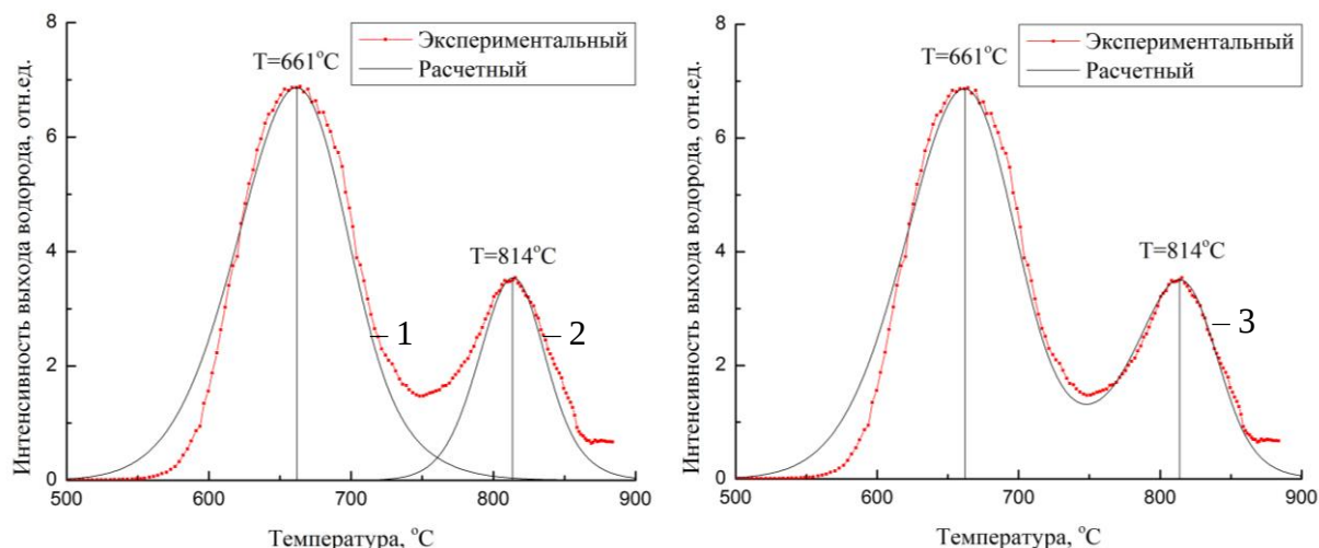
Рисунок 11. Экспериментальные и расчетные зависимости плотности потока водорода термостимулированного газовыделения из Ti, насыщенного водородом по методу Сиверта: 1 – диффузия, 2 – разложение гидрида титана, 3 – диффузия + разложение гидрида титана. Параметры процесса термодесорбции водорода из Ti: d = 0,93 мм, C = 0,33 масс%, D_0 = 10^{-2} \text{ см}^2 \cdot \text{с}^{-1} , E_a = 0,49 эВ, K_0' = 8 \cdot 10^{-9} \text{ см}^4 \cdot \text{с}^{-1} , E_K' = 3,04 эВ, v_0 = 6 \cdot 10^{13} \text{ с}^{-1} , E_{dec} = 3,06 эВ.
