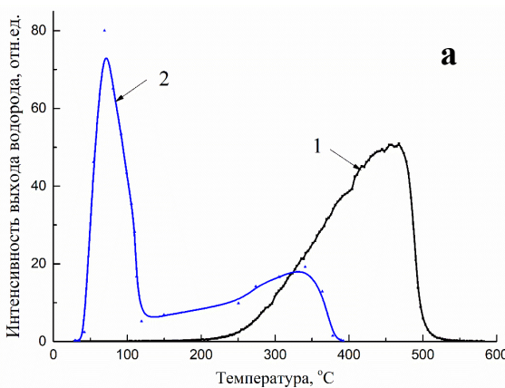
Рисунок 6. Экспериментальные результаты термо- и радиационно-стимулированного газовыделения из Ti, Zr, Ni, Pd. а) Зависимость плотности потока водорода от температуры: 1 – ТСГВ, 2 – РСГВ. б) Экспериментальные результаты процесса РСГВ: 1 – Зависимости плотность потока водорода от времени, 2 – Зависимости температуры от времени.
