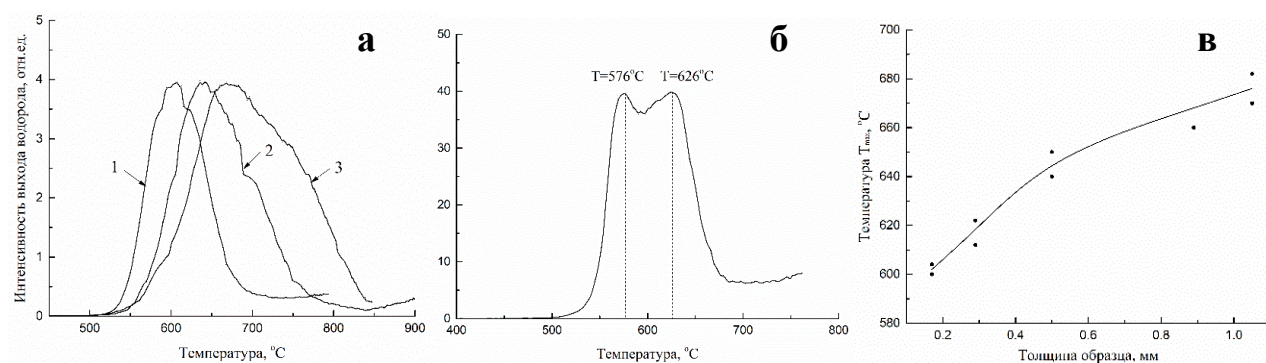
Рисунок 2. Зависимость плотности потока водорода с поверхности пластинок титана (BT1-0) различной толщины при линейном нагреве. Катодное насыщение в \text{H}_2\text{O} + \text{H}_2\text{SO}_4 (1М): а) 1 – 0,17 мм, 2 – 0,5 мм, 3 – 1,05 мм, t = 6 ч, j = 200 мА/см 2 ; б) d = 0,2 мм, t = 24 ч, j = 40 мА/см 2 . Скорость нагрева 1 град/сек; в) Зависимость температуры T_{\text{max}} достижения максимума интенсивности термогазовыделения водорода от толщины образца титана.
