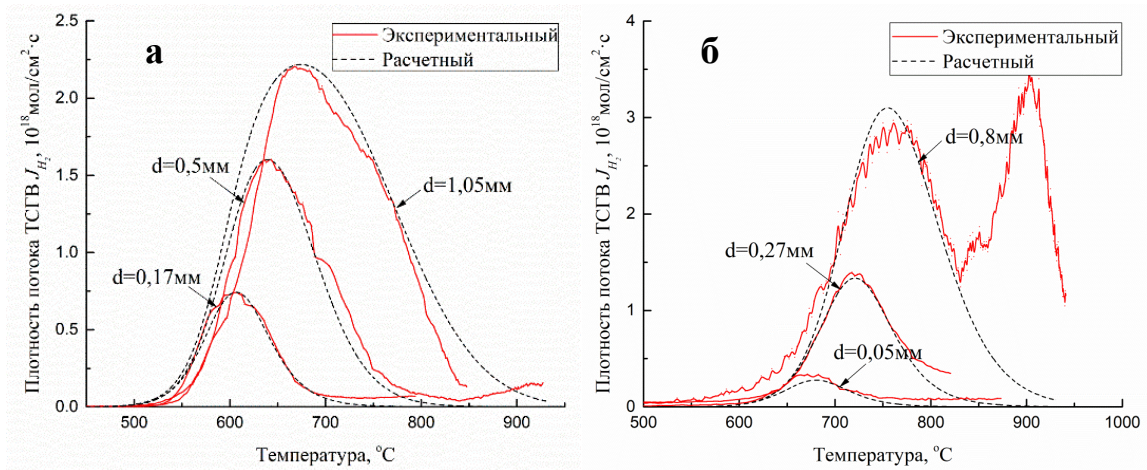
Рисунок 9. Экспериментальные и расчетные зависимости плотности потока водорода термостимулированного газовыделения из пластинок а) Ti: d = 0,17\text{--}1,05 мм, катодное насыщение: t = 6 ч, j = 200 мА/см 2 , \text{H}_2\text{O} + \text{H}_2\text{SO}_4 (1М); б) Zr: d = 0,05\text{--}0,8 мм, катодное насыщение: t = 21\text{--}48 ч, j = 20\text{--}200 мА/см 2 , \text{H}_2\text{O} + \text{H}_2\text{SO}_4 (0,1–1М). Скорость нагрева 1 град/сек.
