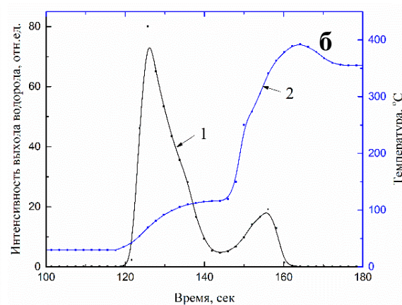
Рисунок 6. Экспериментальные результаты термо- и радиационно-стимулированного газовыделения из Ti, Zr, Ni, Pd. а) Зависимость плотности потока водорода от температуры: 1 – ТСГВ, 2 – РСГВ. б) Экспериментальные результаты процесса РСГВ: 1 – Зависимости плотность потока водорода от времени, 2 – Зависимости температуры от времени.
