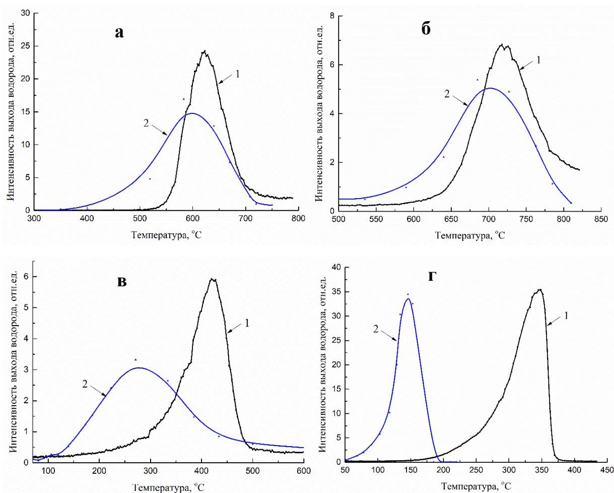
Рисунок 7. Экспериментальные результаты термостимулированного газовыделения водорода и в режиме нагрева переменным током (50Гц) из пластинок Ti, Zr, Ni, Pd. 1 – ТСГВ, 2 – Нагрев переменным электрическим током (джoule тепло).
