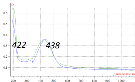
Рис.7 Спектры поглощения PC и PC^+ центров радиационно-окрашенного \gamma -излучением кристалла CaF_2 -10моль.% YF_3 при 300 К: до УФ облучения (зеленый) и после УФ облучения (синий).
