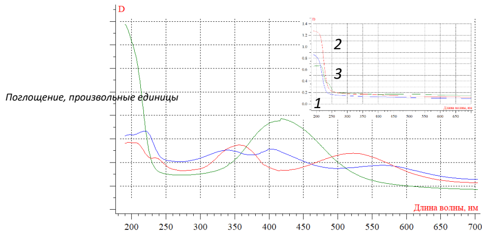
Рис.4 Спектры поглощения \gamma -радиационно-окрашенных кристаллов флюорита: \text{CaF}_2 -красный; \text{CaF}_2 -1моль. \% \text{YF}_3 – синий; \text{CaF}_2 -10моль. \% \text{YF}_3 – зеленый. Условия облучения как на рисунке 8. На врезке приводятся спектры поглощения необлученных образцов \text{CaF}_2 (1), \text{Ca}_{0,99}\text{Y}_{0,01}\text{F}_{2+0,01} (2) и \text{Ca}_{0,90}\text{Y}_{0,10}\text{F}_{2+0,1} (3)
