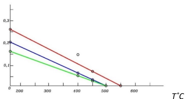
Рис.5 Зависимости температурного изменения коэффициентов поглощения пиков полос ЦО в спектрах кристаллов \text{CaF}_2 (красная), \text{CaF}_2 -1% \text{YF}_3 (синяя) и \text{CaF}_2 -10% \text{YF}_3 (зеленая).
