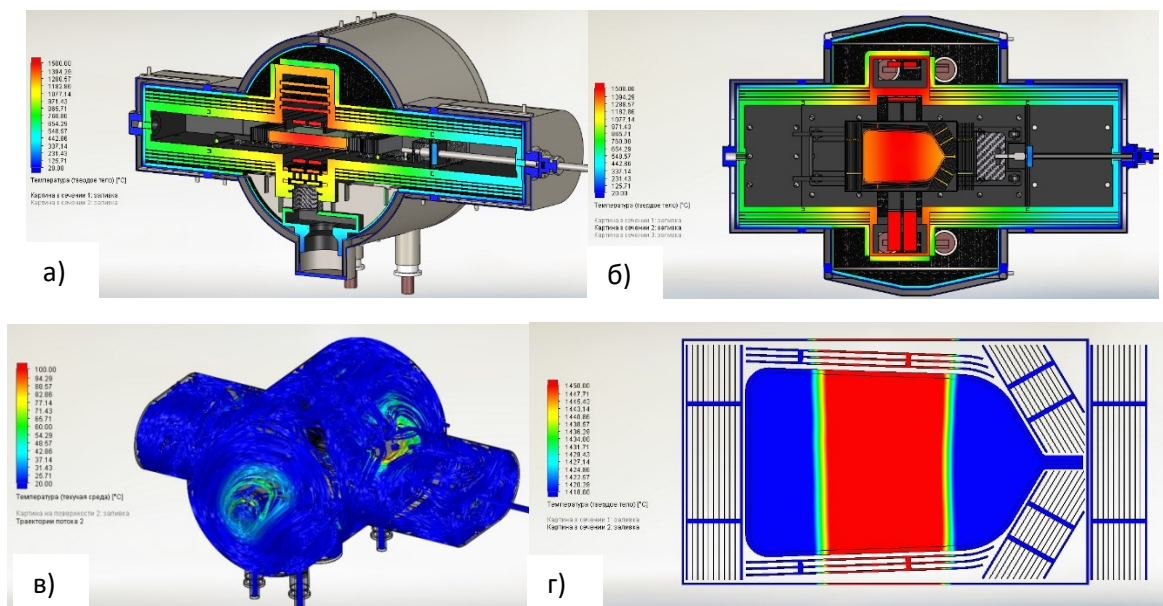
Рис.2. Результаты математического моделирования распределения температуры в твердом теле углиграфитового теплового узла базовой модификации (а, б), в текучей среде (в), в монокристалле \text{CaF}_2 (г), помещенного в кристаллизационный аппарата «Рубитек-1»
