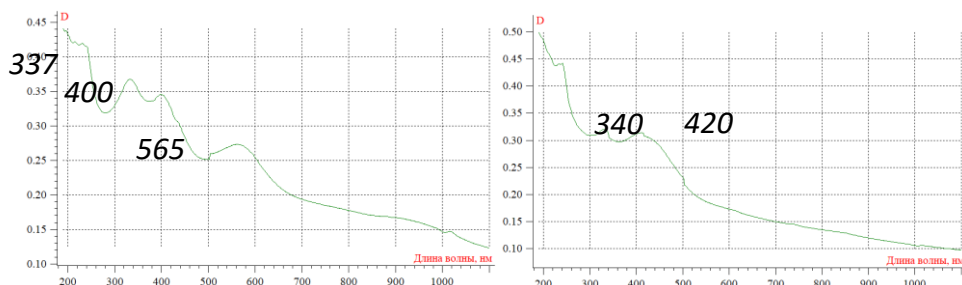
Рис.6 Спектры поглощения PC и PC^+ центров радиационно-окрашенного \gamma -излучением кристалла CaF_2 -1моль.% YF_3 при 300 К: (а)- до УФ облучения; (б)- после УФ облучения.
