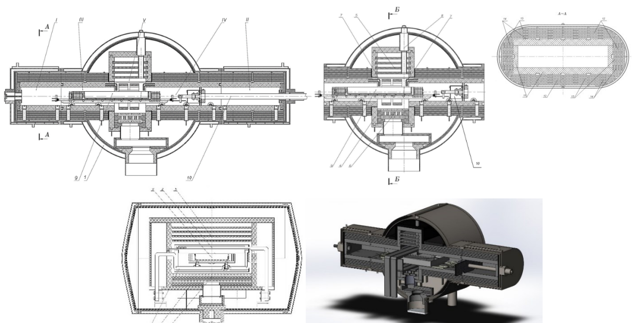
Рис. 1. Базовая компоновочная схема основной конструкции углеграфитового теплового узла, помещенного в кристаллизационный аппарат, где римскими цифрами обозначены: I – загрузочный модуль, II – приемный модуль, III – коридор загрузочного модуля, IV – коридор приемного модуля, V – центральный модуль; арабскими обозначены: 1 – водоохлаждаемый стальной корпус кристаллизационного аппарата, 2 – верхний нагреватель Г-образной формы, 3 – нижний нагреватель перевернутой П-образной формы, 4 – внешний графитовый теплоизоляционный кожух, 5 – верхняя секция внутренних графитовых тепловых экранов, 6 – нижняя секция внутренних графитовых тепловых экранов, 7 – диафрагмы, 8 – смотровое окно, 9 – графитовый тигель с набором тепловых экранов, контейнером и рамой, 10 – механизм горизонтального перемещения, 11 – внутренний графитовый кожух, 12 – внешние сборно-разборные графитовые теплоизолирующие кассеты, 13 – тепловые экраны, 14 – теплоизолирующие проставки.
