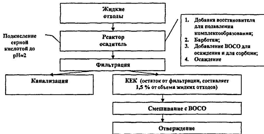
Рис 4. Схема проведения процесса ступенчатой иммобилизации опасных примесей Полигона «Красный Бор»
