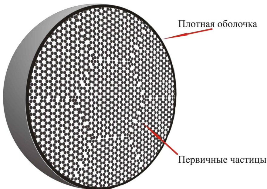
Рисунок 1. – Строение микросфер \text{SiO}_2\text{-TiO}_2 и \text{TiO}_2 , полученных перексо-методом
