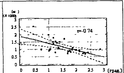
Рис. 6. График линейной модели, аппроксимирующей зависимость длины линий тока от угла наклона
