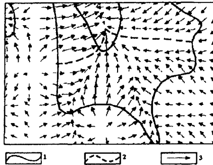
Рис. 1. Траектория движения при вычислении расстояний от узла сетки до горизонтали (линия вдоль векторов), где 1- горизонтали, 2 – траектория, 3- вектора градиентов
