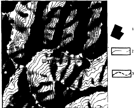
Рис 2 Фрагмент ЦМР, построенной кубическими параболоми по горизонталям топографической карты масштаба 1:200000 (источник света помещен в левый верхний угол): 1- населенные пункты, 2- горизонталы (сечение 20 м); 3 – реки.
