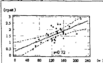
Рис. 5. График линейной модели, аппроксимирующей зависимость угла наклона от абсолютной высоты
