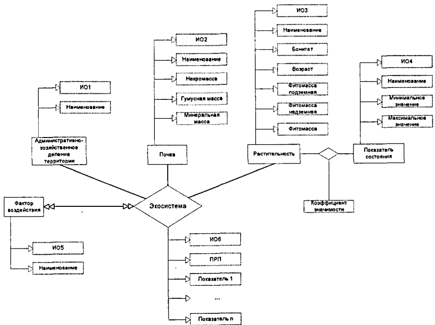
Рисунок 1. Концептуальная модель БД
