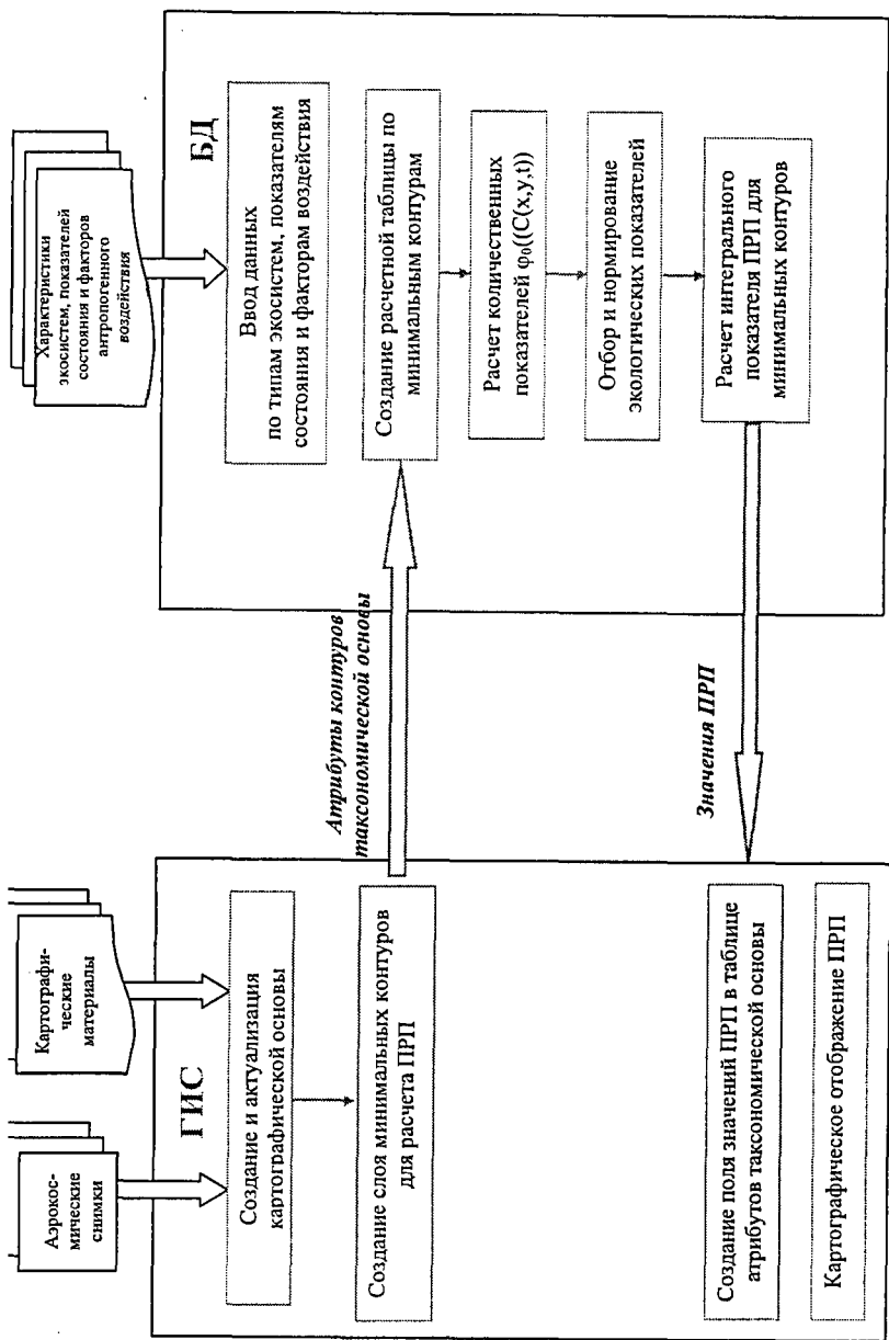
Рисунок 3. Схема взаимодействия специализированной БД и ГИС
